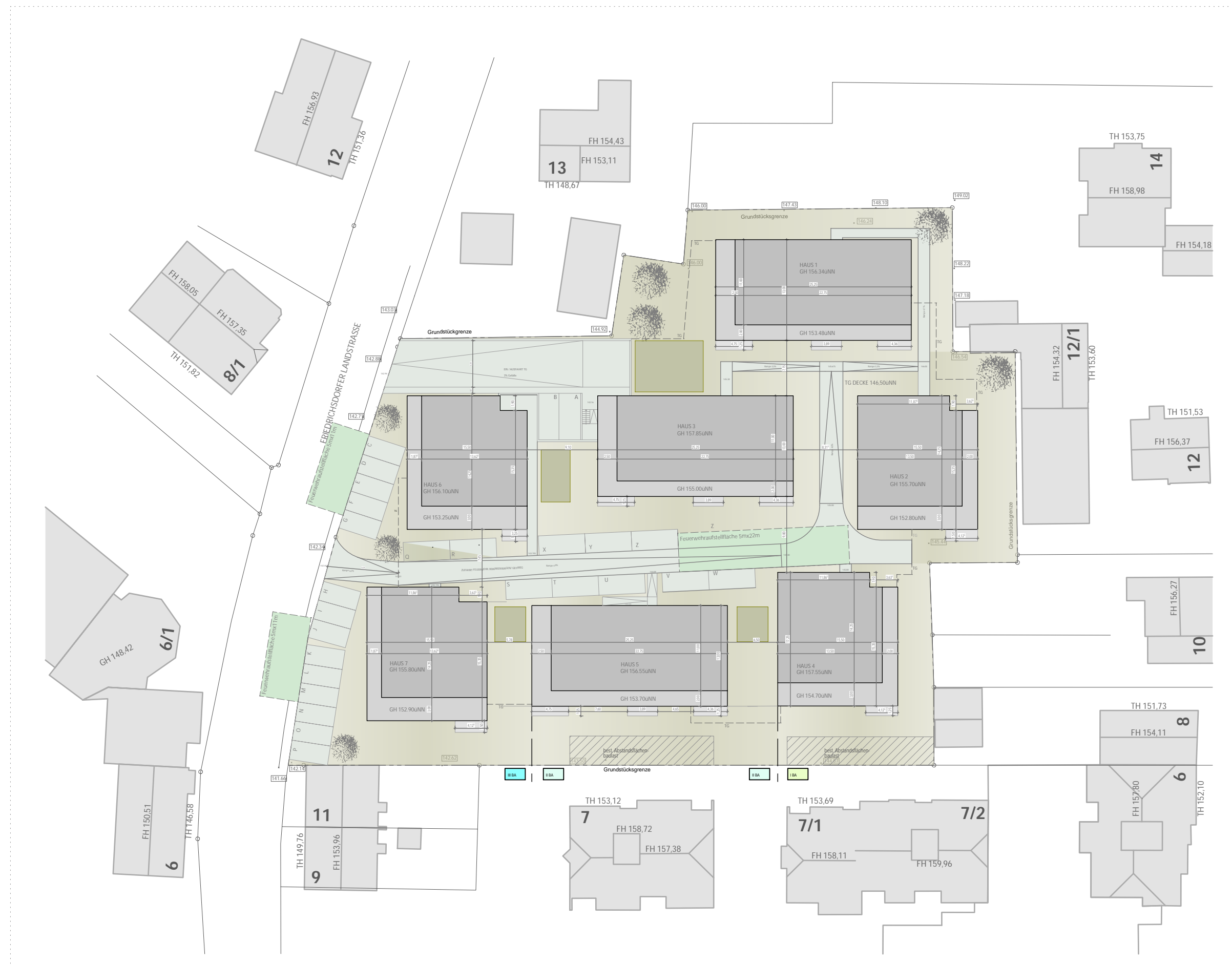
LAGEPLAN M 1:500
